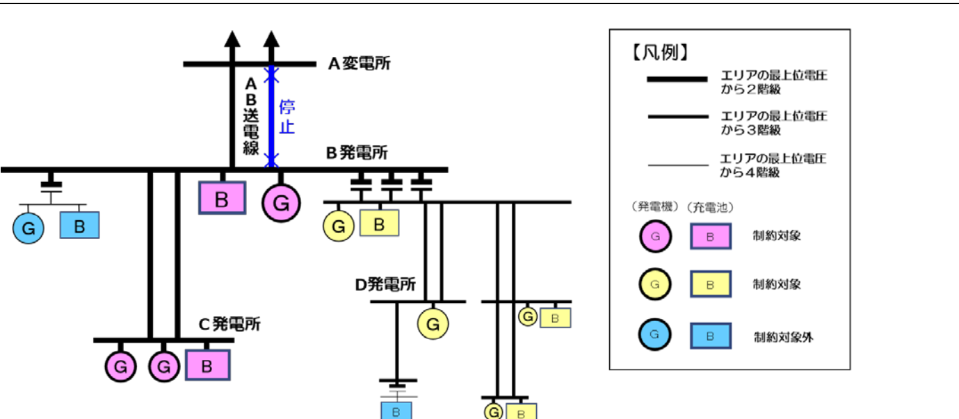
図 3.1-3 発電等制約の対象となる発電設備等の選定例
