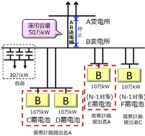
図 3.4-9 N-1 制御対象蓄電池を含む系統における充電制約の振替例
