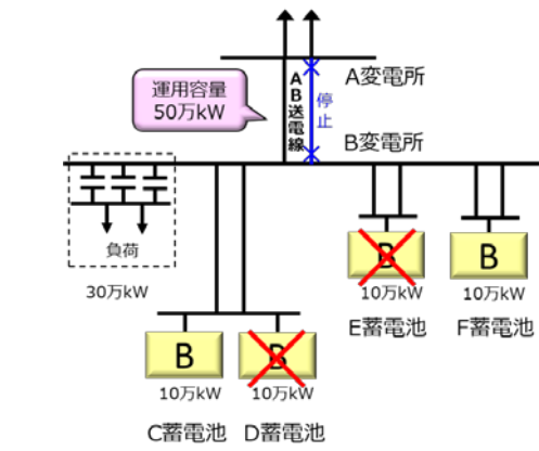
図 3.4-2 発電設備等の作業停止のため充電制約量を配分しない例
