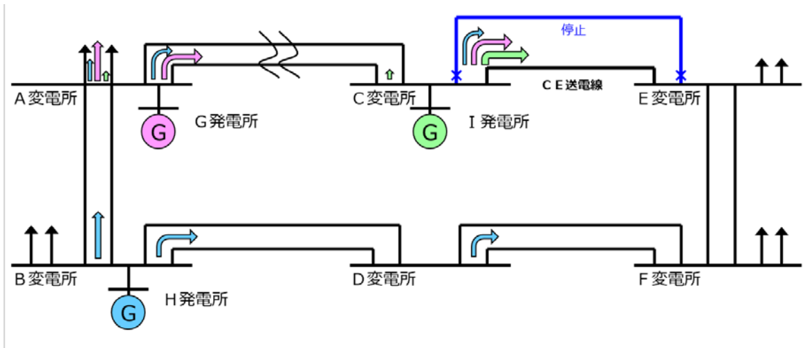
図 3.3-15 ループ系統における発電制約効果
