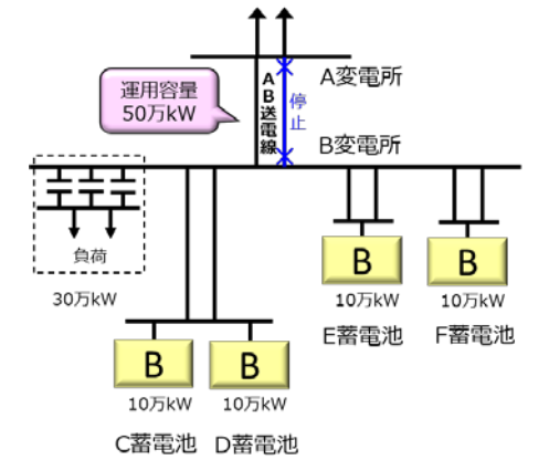
図 3.4-1 蓄電池の作業停止がなく定格容量比率按分で充電制約量を配分する例
