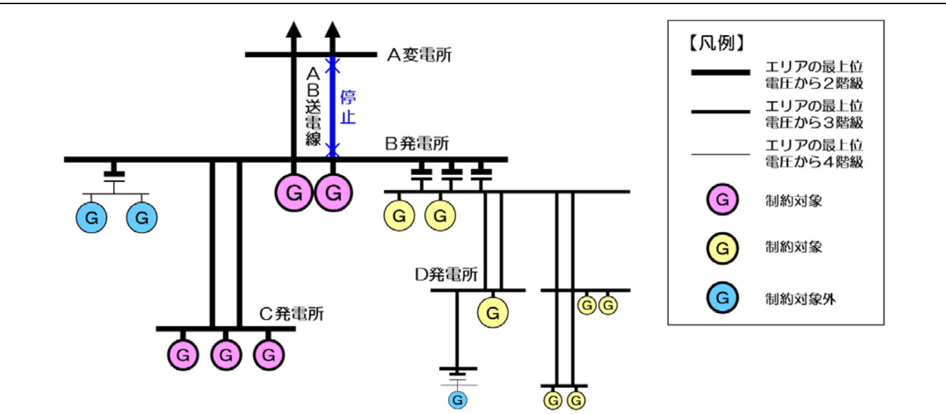
図 3.1-2 発電制約の対象となる発電設備等の選定例
