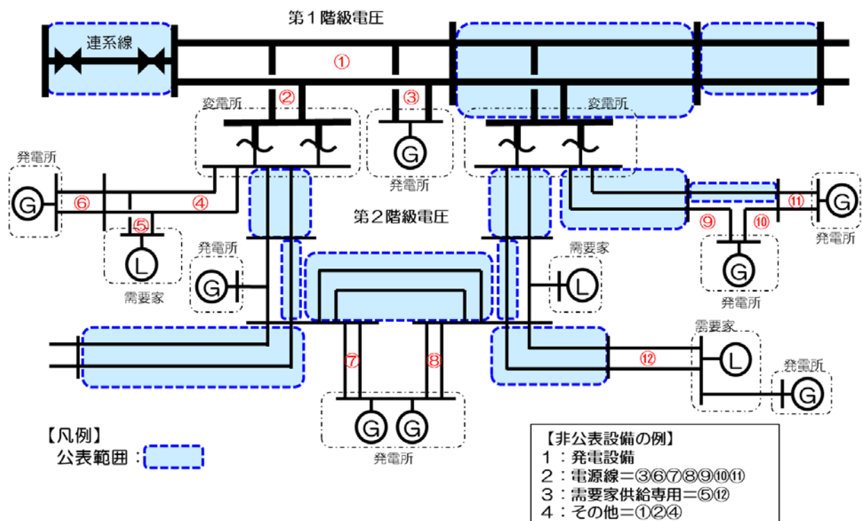
図 2.7-1 作業停止計画の公表範囲の例
