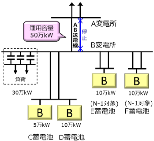
図 3.4-6 N-1 制御適用蓄電池が複数ある場合の定格容量比率按分の例
