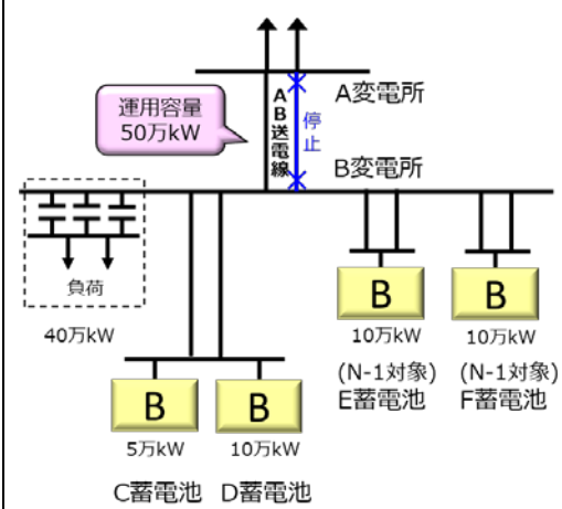
図 3.4-7 N-1 制御適用蓄電池の充電制約だけでは充電制約が解消しない場合の 定格容量比率按分の
