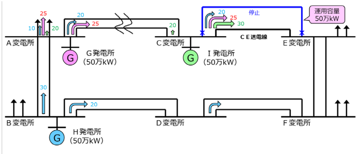
図 3.3-16 ループ系統における発電制約効果の例
