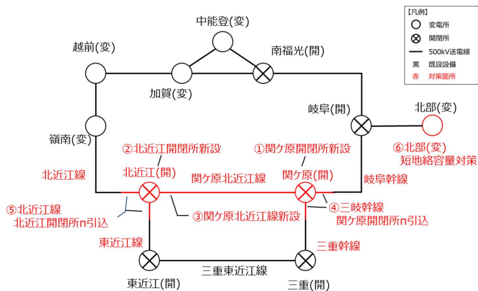
図 工事概略図
