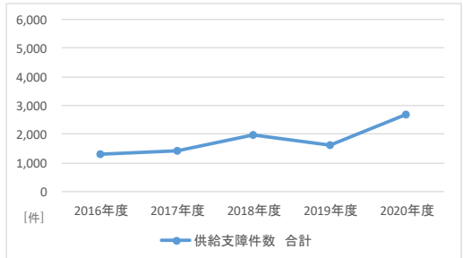
図15 (九州、2016～2020年度)事故発生箇所別供給支障件数
