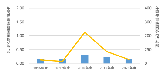
図19 (全国、2016～2020年度) 低圧電灯需要家停電実績
