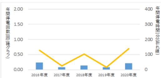
図28 (九州、2016～2020年度) 低圧電灯需要家停電実績
