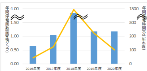
図29 (沖縄、2016～2020年度) 低圧電灯需要家停電実績
