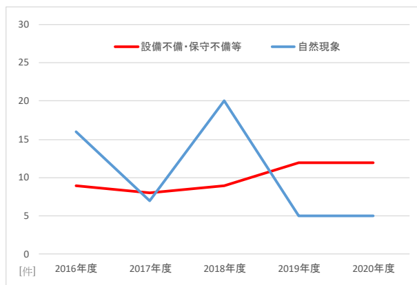
図 18 (全国、2016～2020年度) 供給支障原因
