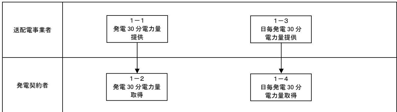
図2-1 業務フロー
