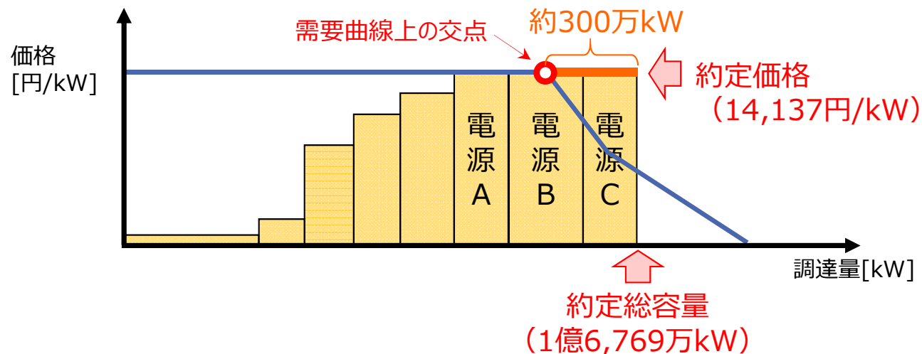
今回の約定結果
