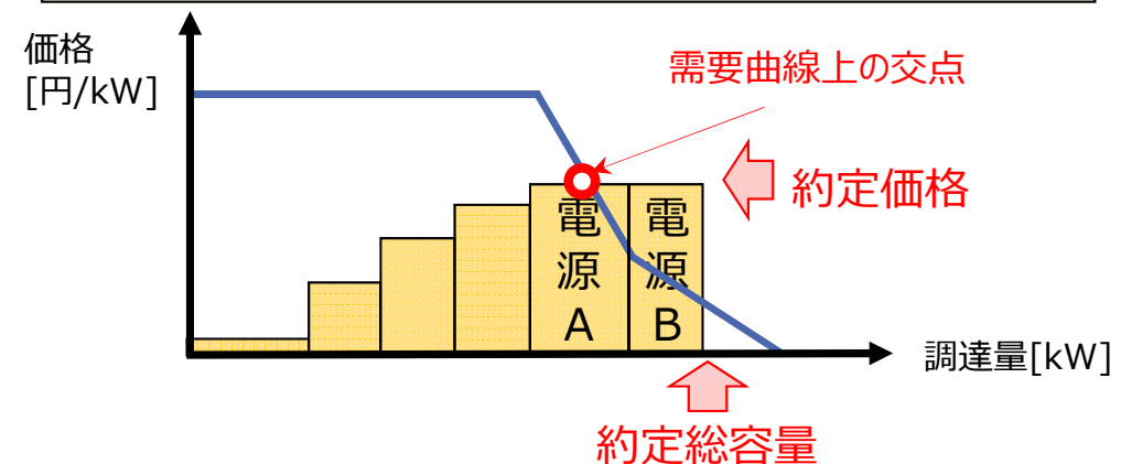
約定価格で応札した電源が複数の場合の例
