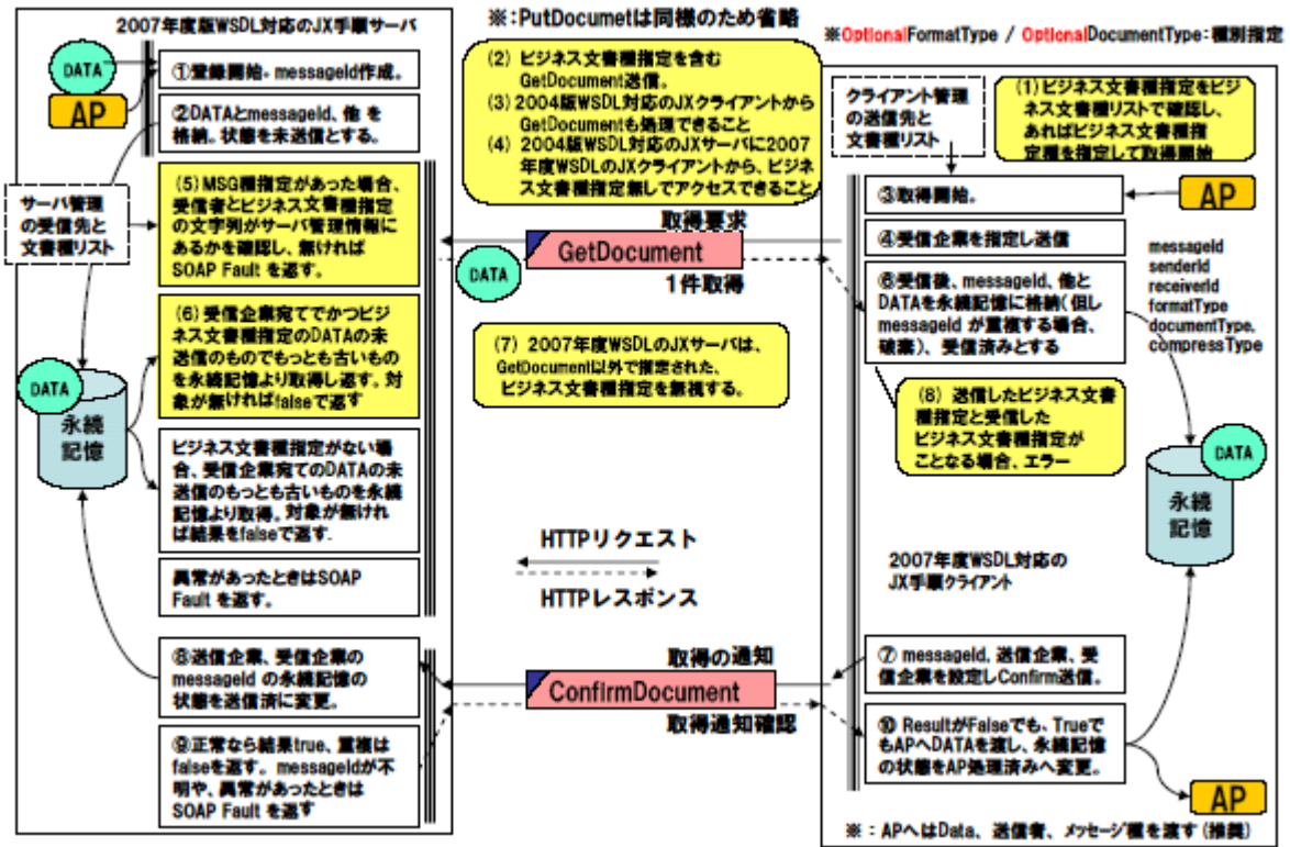
図 3-11 JX 手順動作フロー
