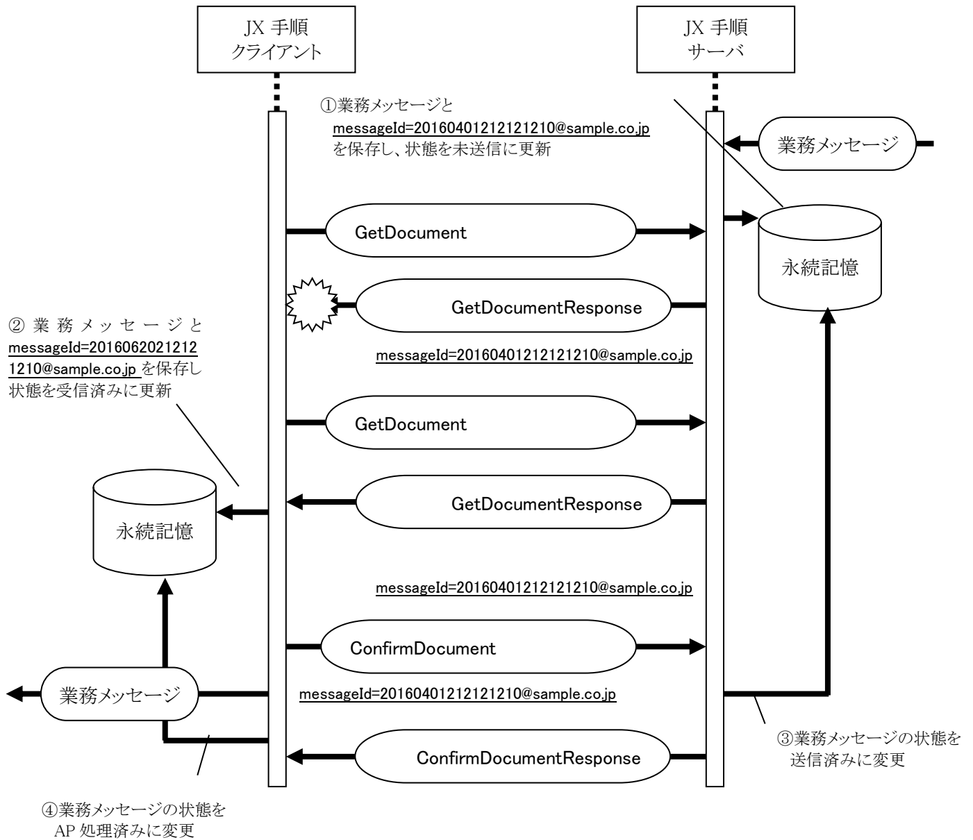
図 3-8 業務メッセージ受信時の欠落防止
