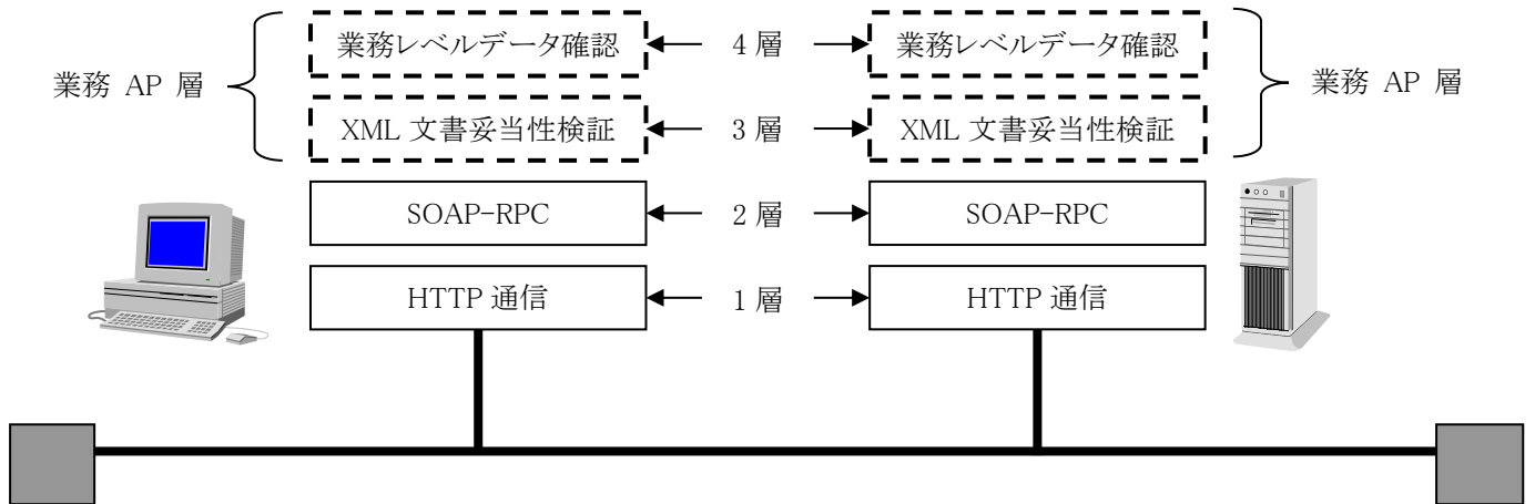
図 3-12 階層別エラーの考え方
