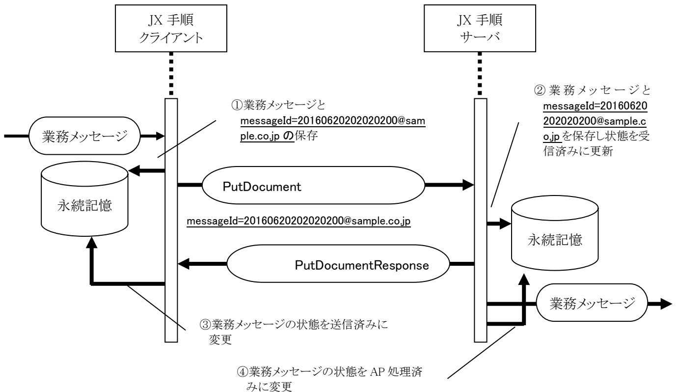
図 3-3 JX 手順レベルの送信シーケンス
