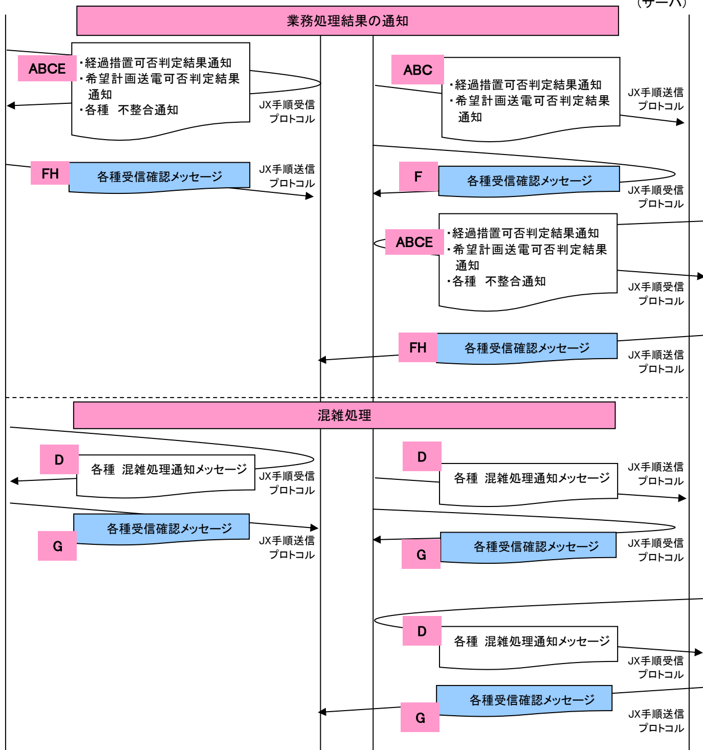
図 4-2 発電計画等伝送フロー(2)
