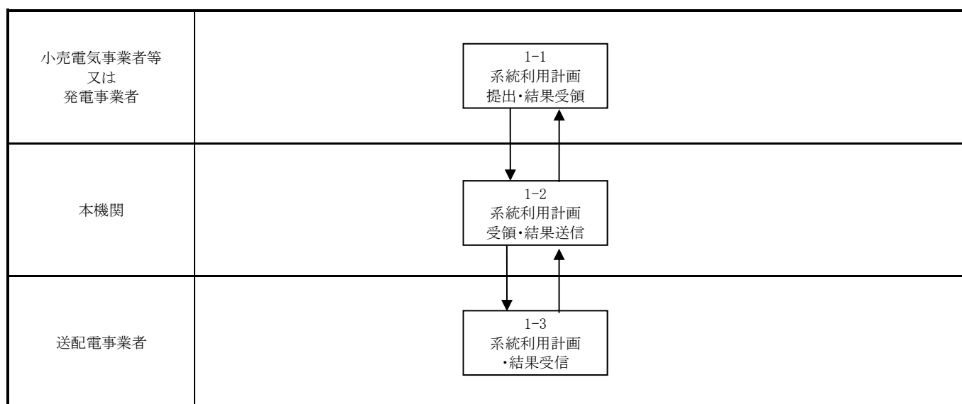
図 2-1 業務フロー
