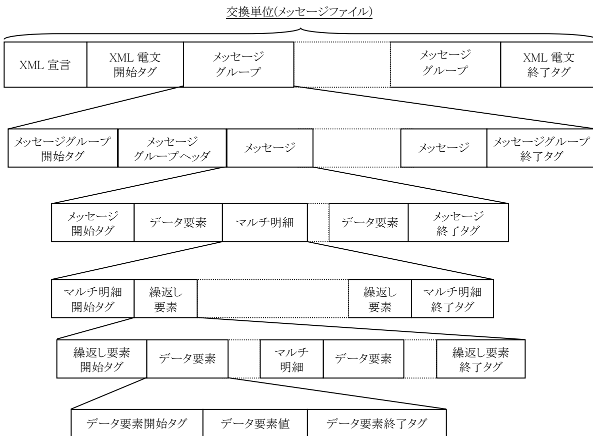
図 4-12 XML 電文の階層構造
