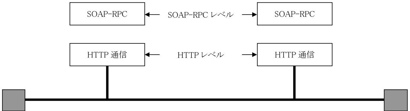
図 3-2 JX 手順通信レイヤ構造
