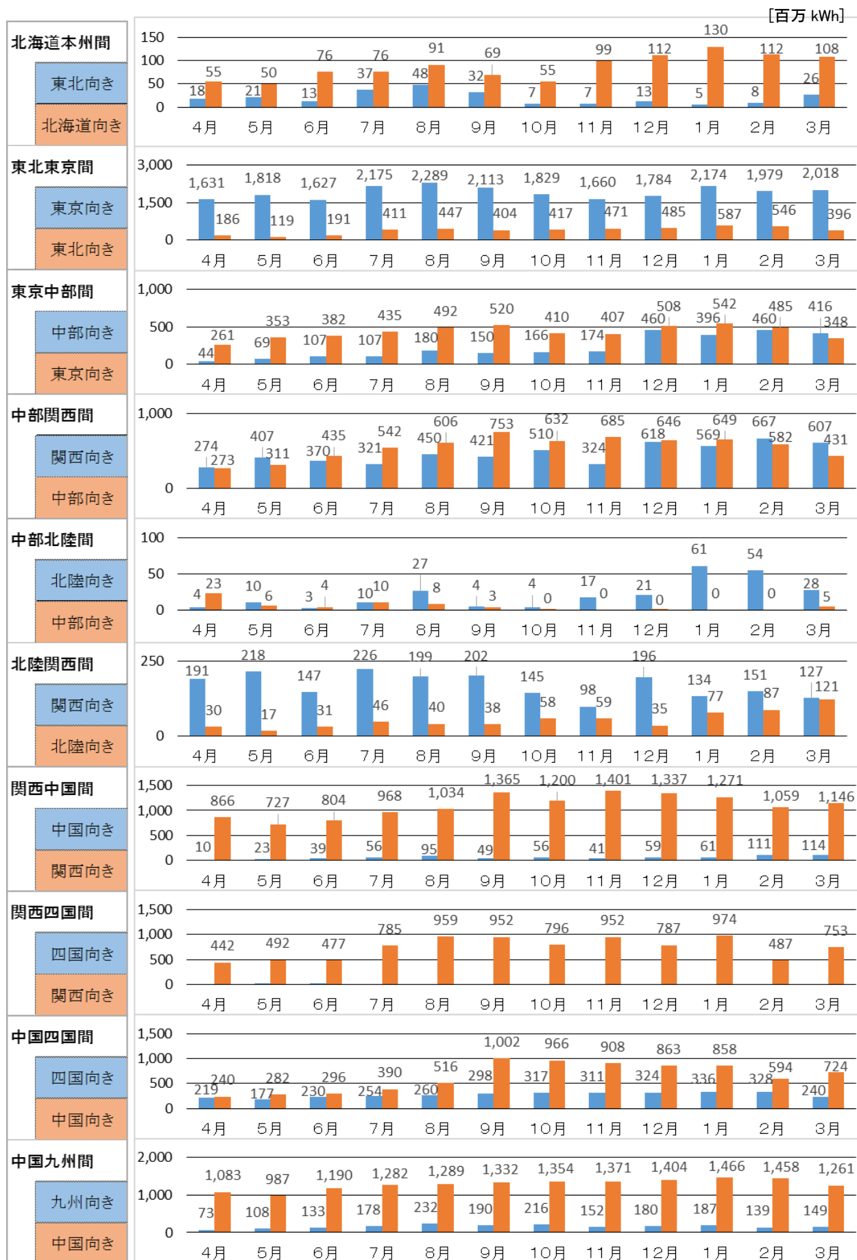
図 2-4 月別連系線利用状況（平成 28 年度）
