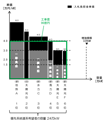
〔系統連系順位の決定イメージ〕
