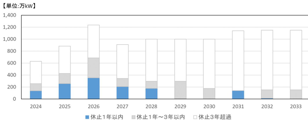
図2-7 火力休止電源の状況
