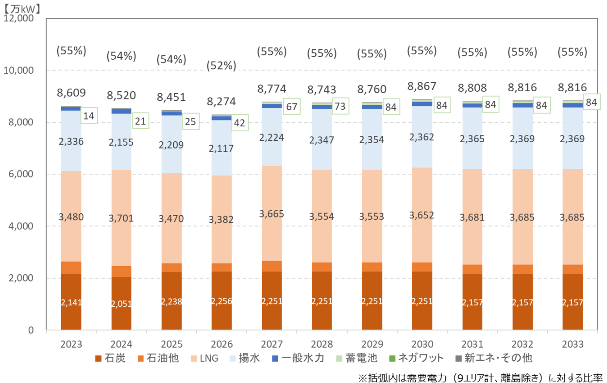
図3-5 調整能力の推移
