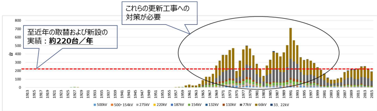
図４－５ 変圧器の物量分布（66kV（一部 22kV）～500kV）
