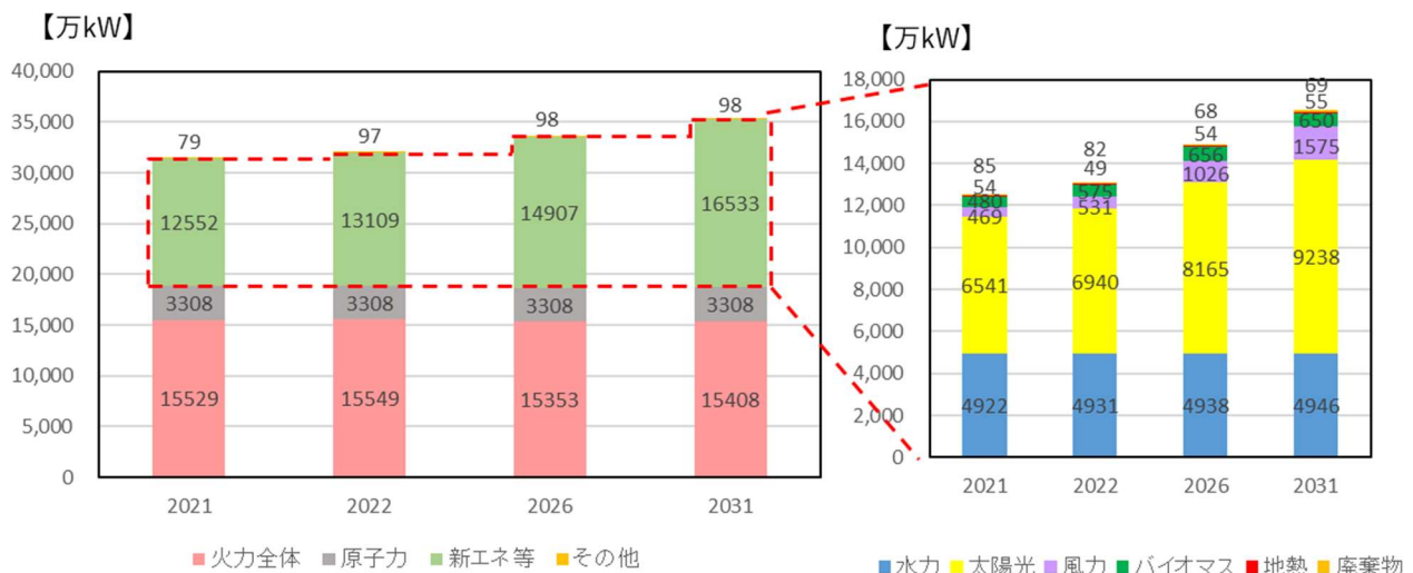
図 3－1 設備容量（全国合計）
