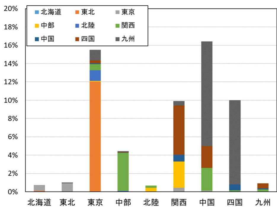
図 5－4 エリア外調達電力量比率
