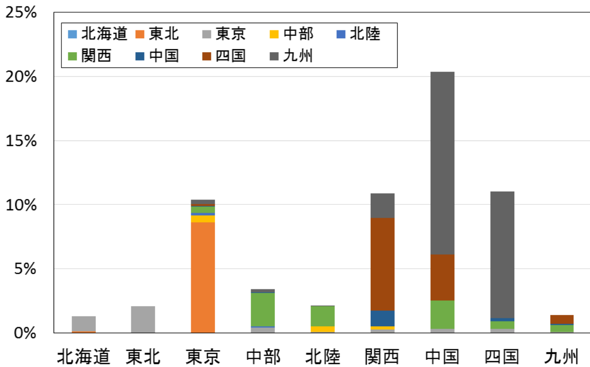
図5-4 エリア外調達電力量
