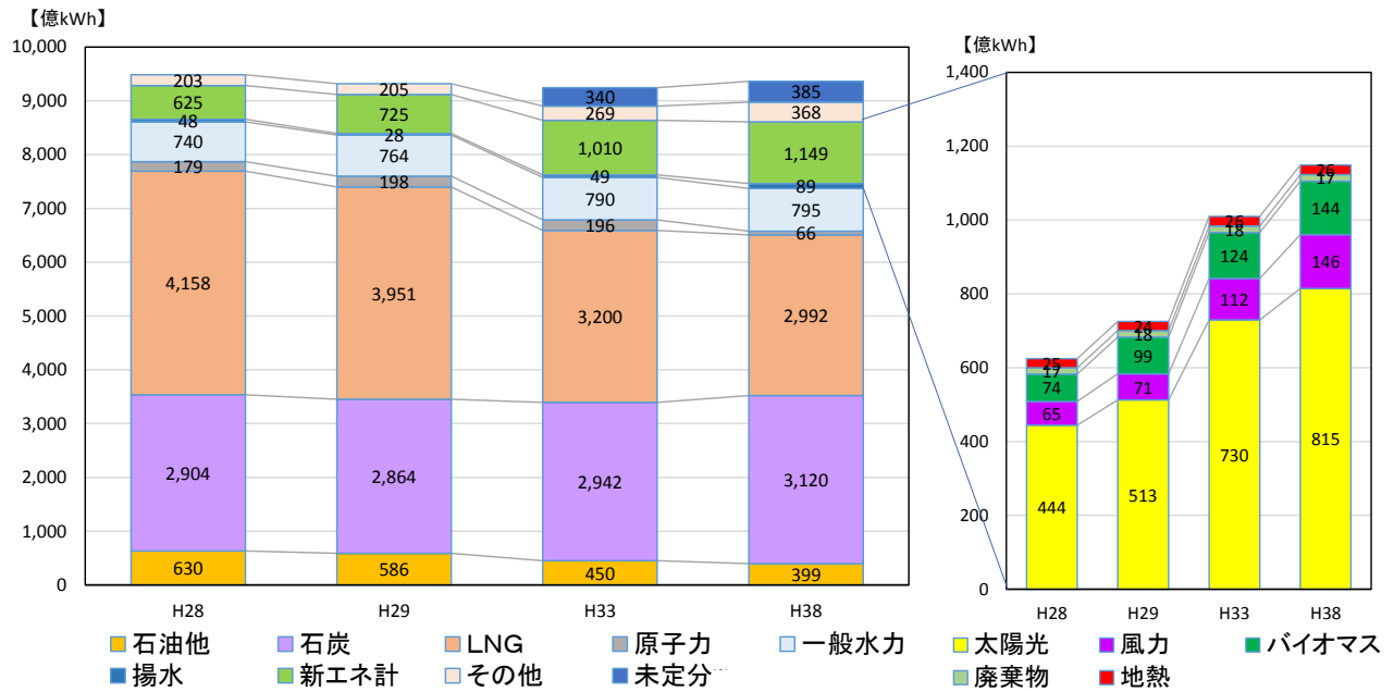
図 3 - 3 電源別発電電力量の推移 (全国合計)
