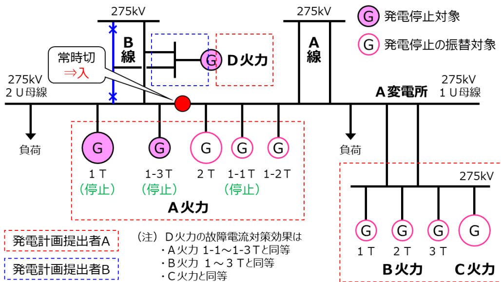
図 3.3-19 故障電流対策のための発電機停止の振替例
