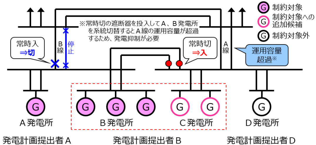
図 3.3-21 系統切替を伴う流通設備作業停止時の発電制約対象範囲
