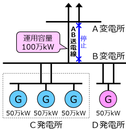
図 3.3-1 発電機の作業停止がなく定格容量比率按分で発電制約量を配分する例
