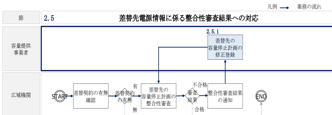
図 2-26 差替先電源情報に係る整合性審査結果への対応の詳細構成
