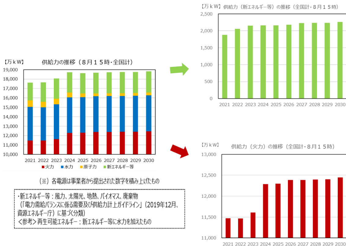
図2-13 電源別供給力の推移
