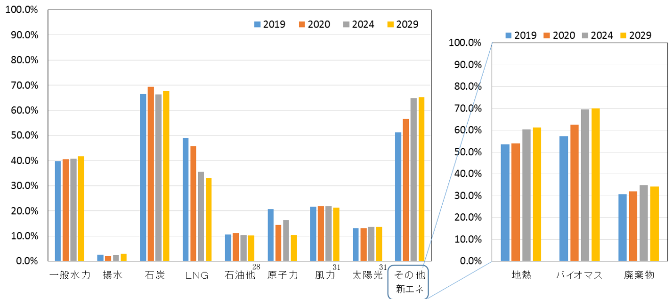
図 3－5 設備利用率の推移（全国合計）
