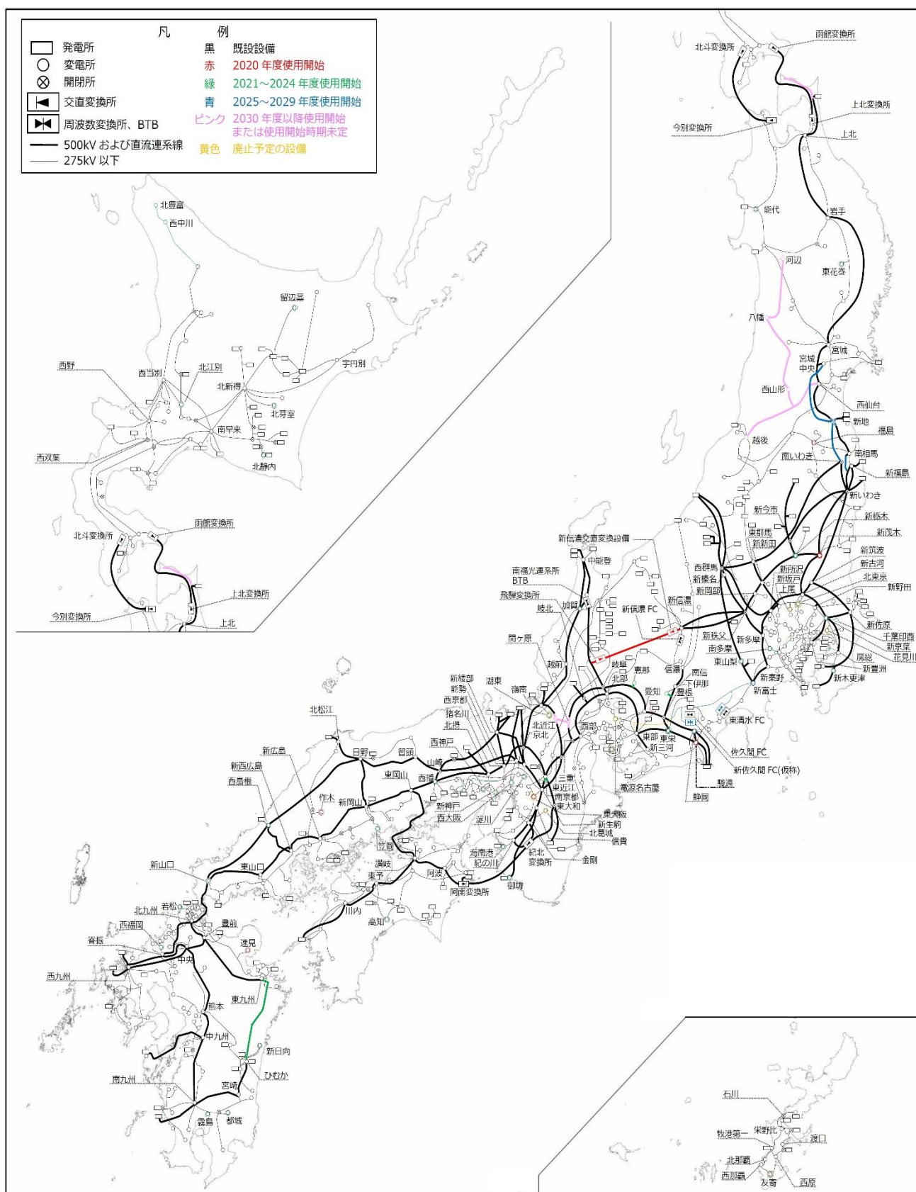
図 4 - 1 電力系統の状況
