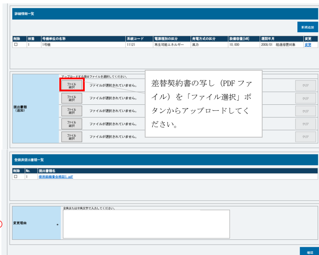
図 3-8 「電源等情報変更申込画面」の画面イメージ
