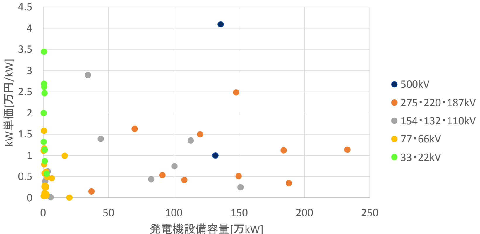
電源が接続する電圧階級別のネットワーク増強工事实績
