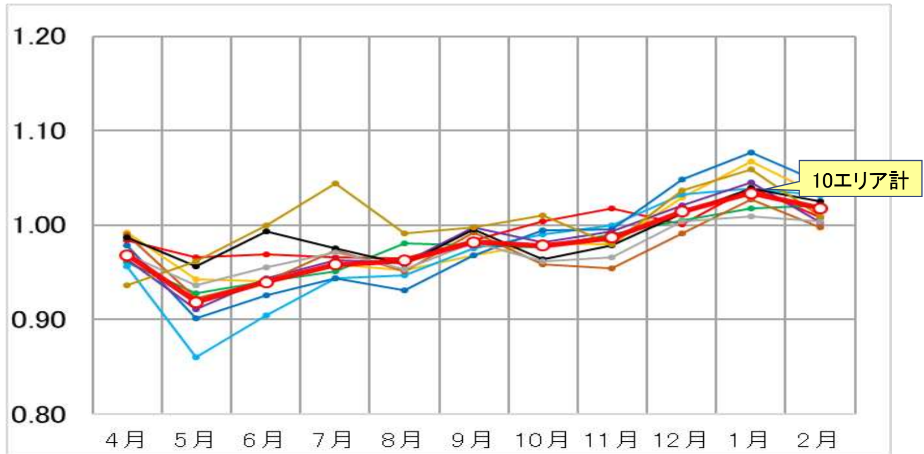
【図1】送電端電力量（気象補正後、前年同月比）
