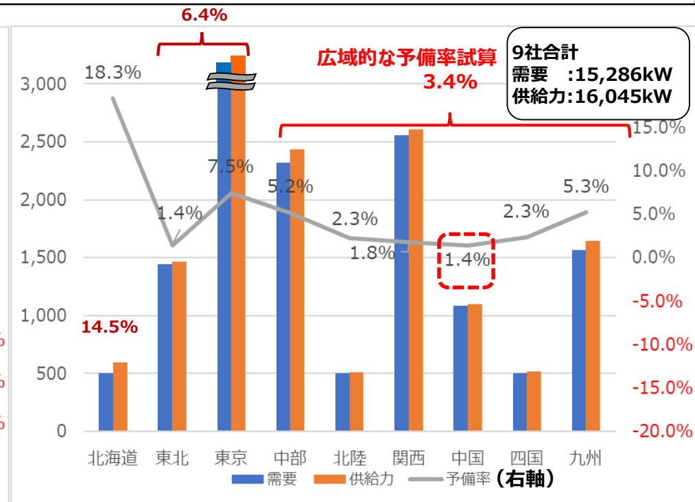
図2.エリア予備率他（実績）
