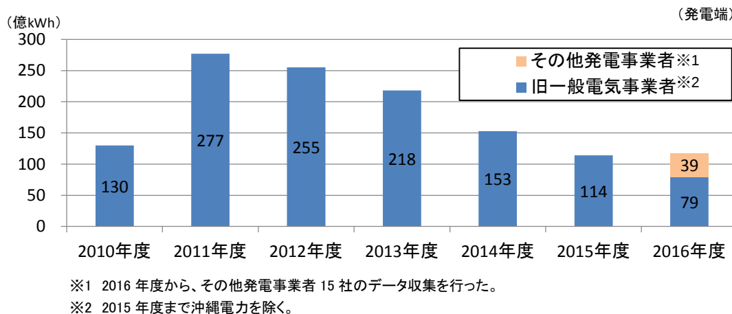
【図 2 老朽火力の冬季（12～2 月）発電電力量推移】
