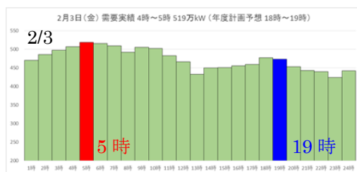
【図 1 需要実績ロードカーブ（北海道、中国エリア）】
