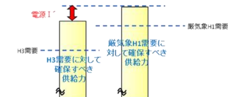
【図 5 電源Ⅰ' の必要量】 10
