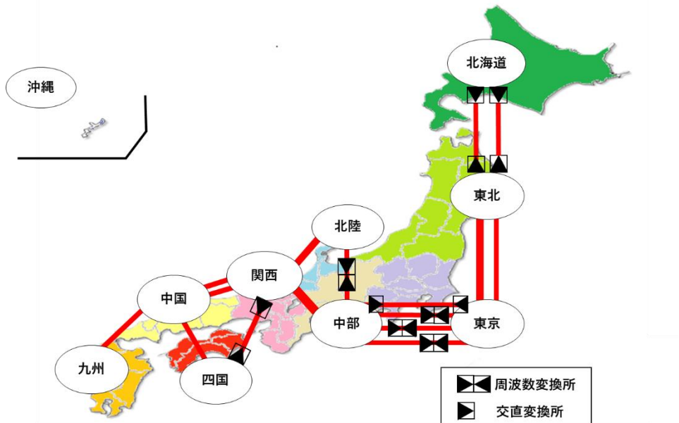
図2-1 連系線
