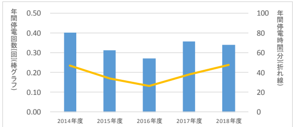
図30 (四国、2014~2018年度) 低圧電灯需要家停電実績
