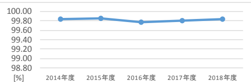
図3 (東地域、2014～2018年度)0.1Hz以内周波数時間滞在率
