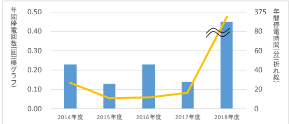
図26 (中部、2014~2018年度) 低圧電灯需要家停電実績
