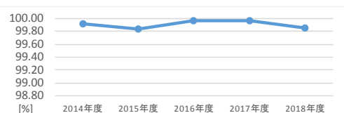
図2 (北海道、2014～2018年度)0.1Hz以内周波数時間滞在率
