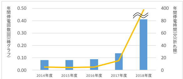
図28 (関西、2014~2018年度) 低圧電灯需要家停電実績
