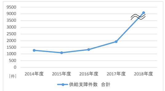
図15 (関西、2014～2018年度)事故発生箇所別供給支障件数
