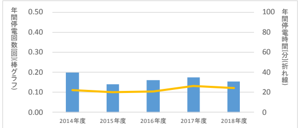
図27 (北陸、2014~2018年度) 低圧電灯需要家停電実績
