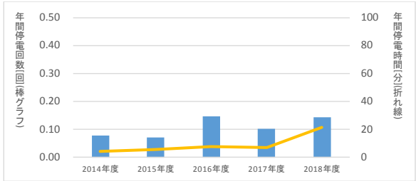
図25 (東京、2014~2018年度) 低圧電灯需要家停電実績
