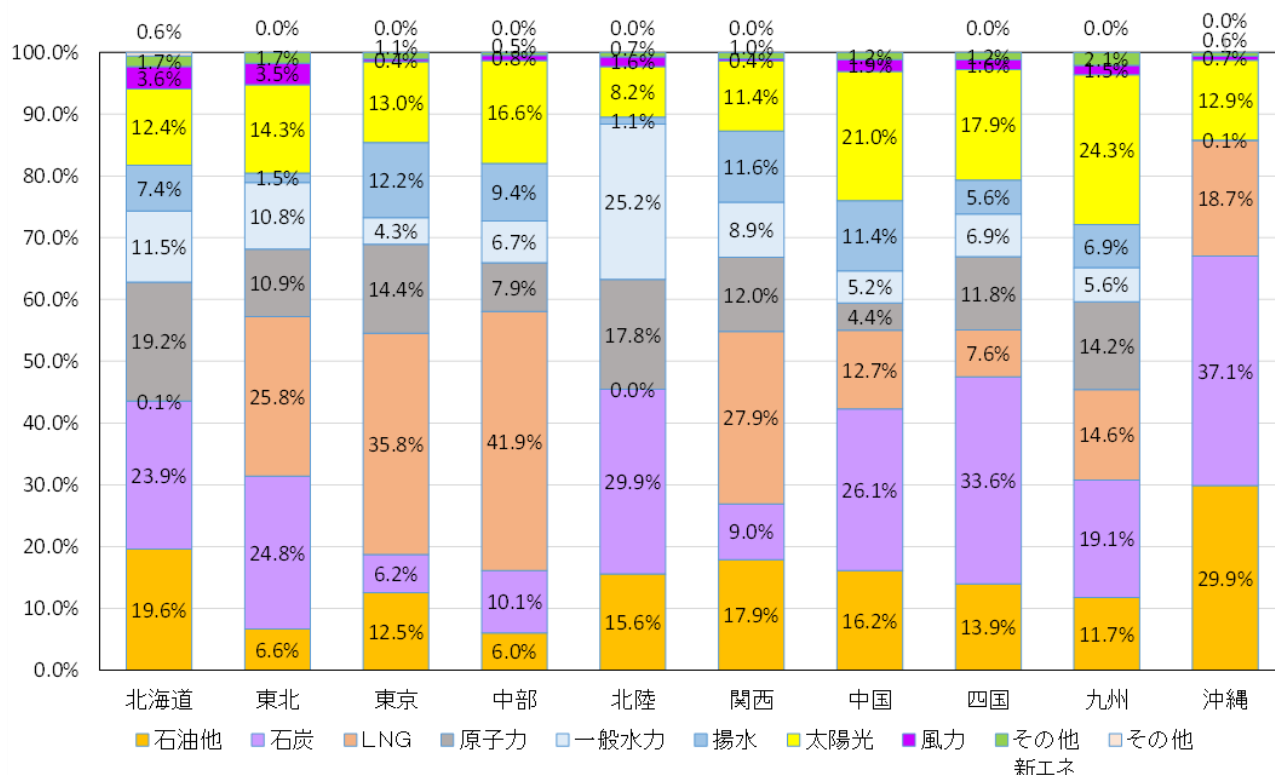
図３－６ ２０１７年度末のエリア別の電源（kW）構成比
