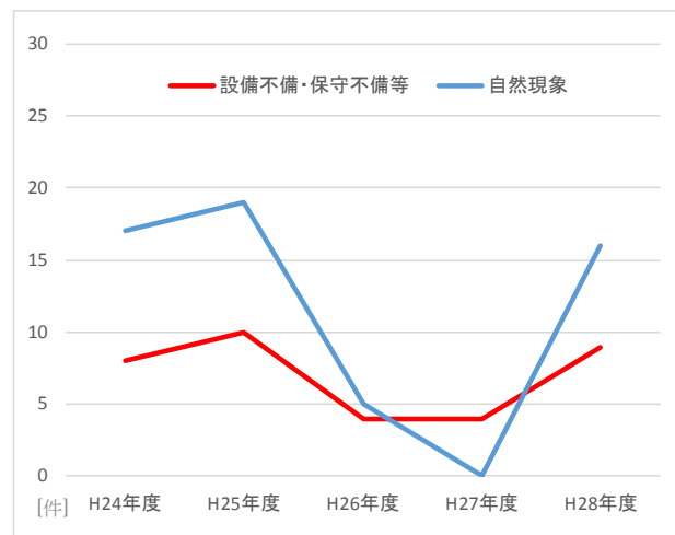
図24 (全国、平成24～28年度) 供給支障原因
