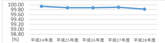
図3 (東北、平成24～28年度)0.1Hz以内周波数時間滞在率
