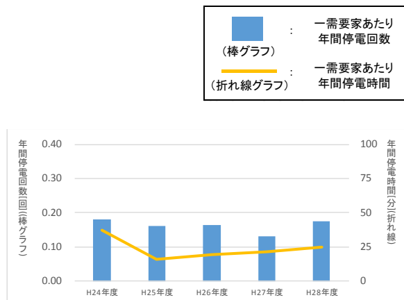
図25 (全国、平成24～28年度) 低圧電灯需要家停電実績
