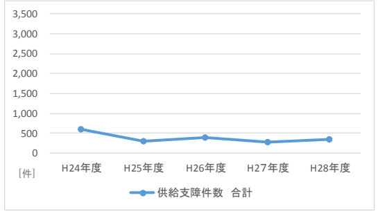
図17 (北陸、平成24～28年度)事故発生箇所別供給支障件数
