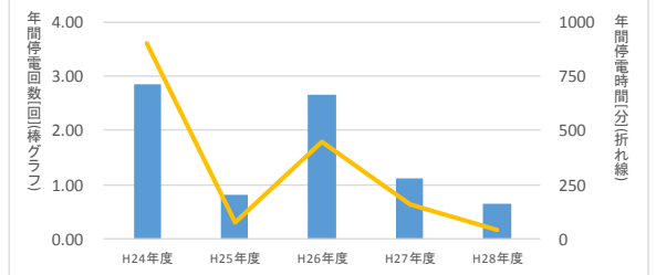
図35 (沖縄、平成24～28年度) 低圧電灯需要家停電実績
