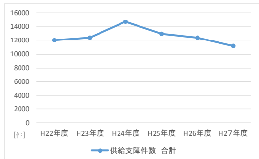
図12 (全国、平成22～27年度)事故発生箇所別供給支障件数
