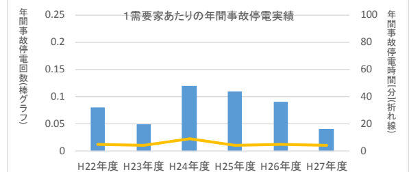
図29 (北陸、平成22～27年度) 需要家停電実績
