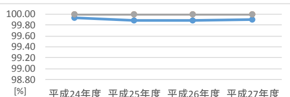
図3 (東北、平成24～27年度) 周波数時間滞在率)
