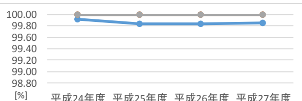
図4 (東京、平成24～27年度) 周波数時間滞在率)
