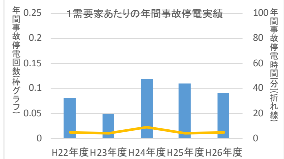
図26 (北陸、平成22～26年度) 需要家停電実績
