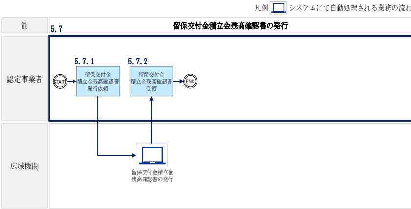
図 5-11 交付金相当額積立金残高確認書の発行の詳細構成
