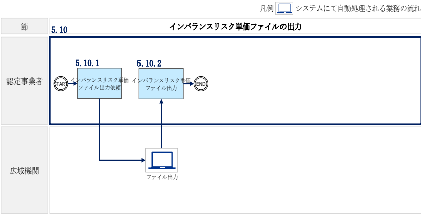
図 5-18 インバランスリスク単価ファイルの出力の詳細構成
