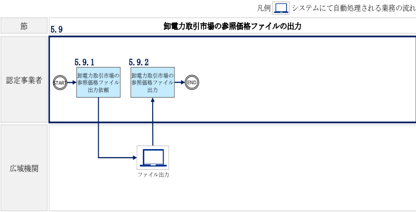
図 5-15 卸電力取引市場の参照価格ファイルの出力の詳細構成
