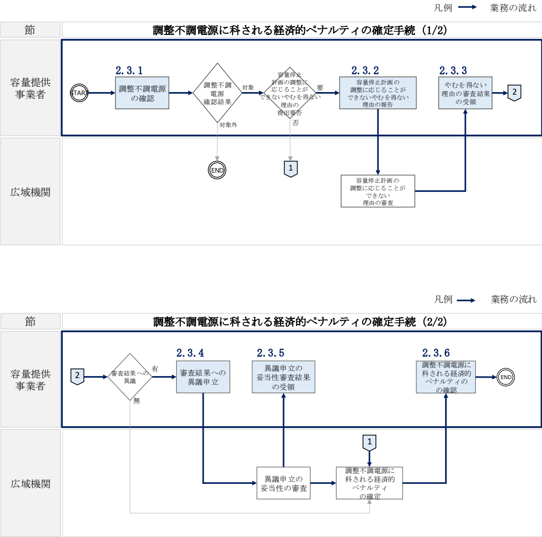
図 2-27 調整不調電源に科される経済的ペナルティの確定手続の詳細構成
