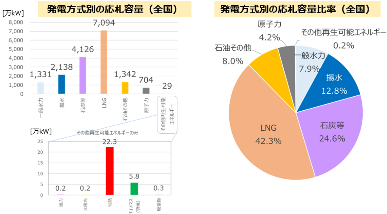
図 4 発電方式別の応札容量と比率
