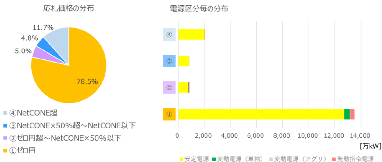
図 6 応札価格の分布
