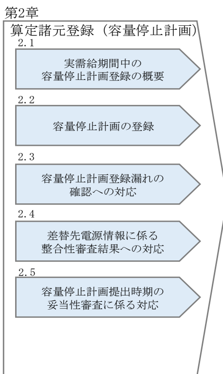
図 2-1 第2章の構成
