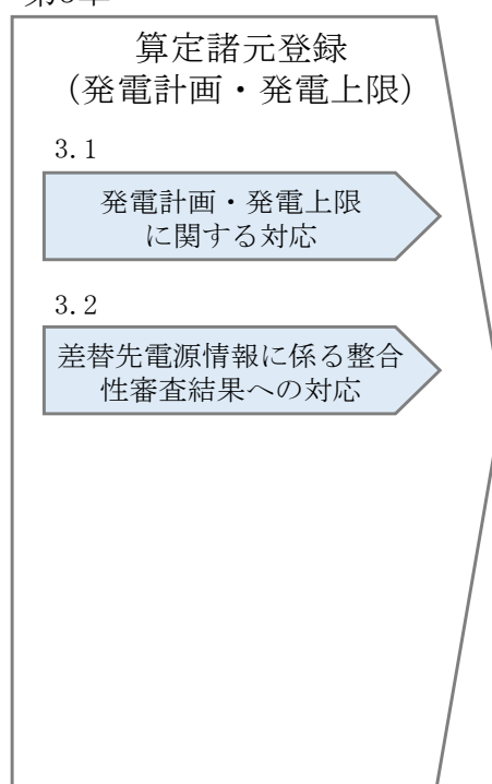
図 3-1 第3章の構成
