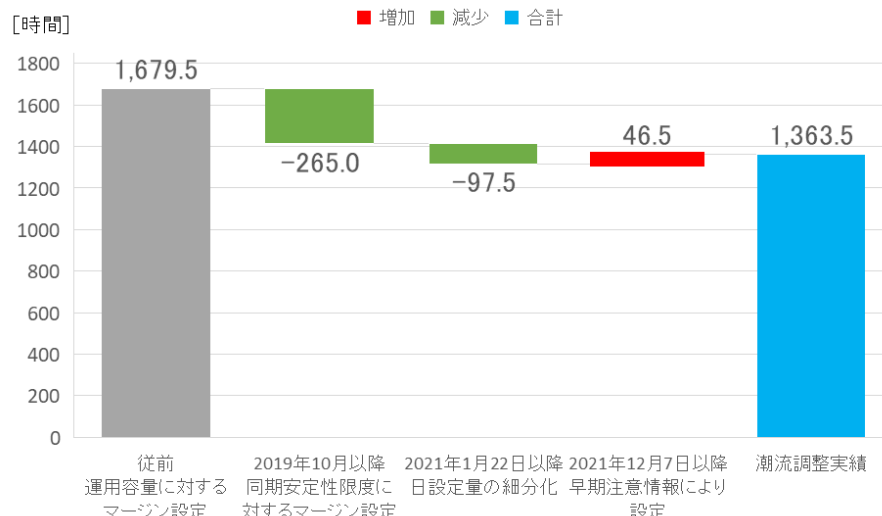
マージン設定に関する一部運用見直しによる 潮流調整時間抑制実績
