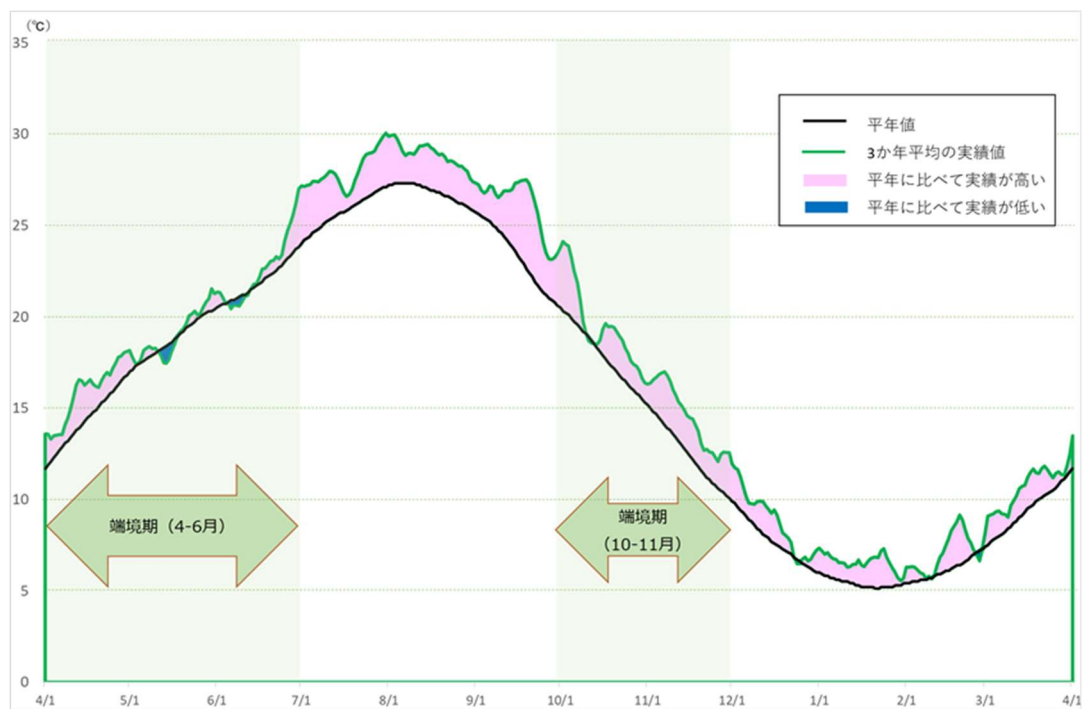
添付図 7-5 日平均気温の推移（東京）
