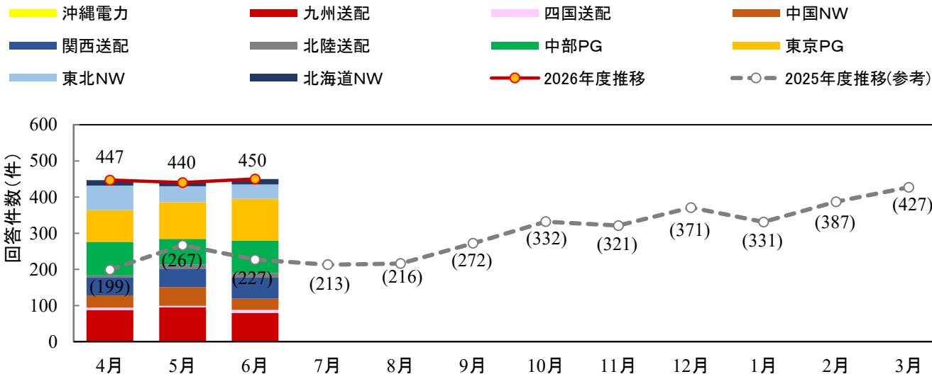
図19 契約申込み 回答件数(一般送配電事業者合計) [2026年度4月～6月]
