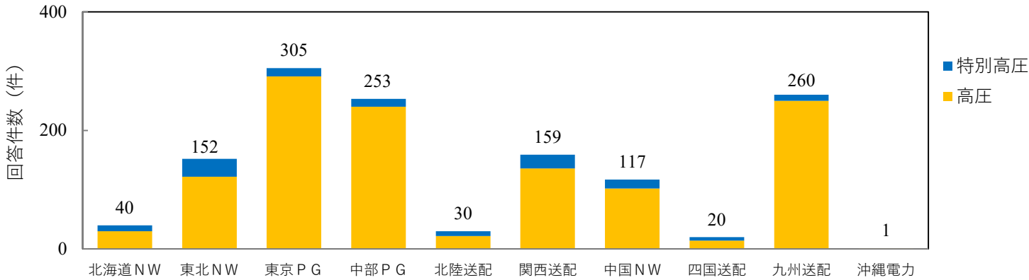
図18 契約申込み 回答件数(一般送配電事業者別) [2026年度4月～6月]
