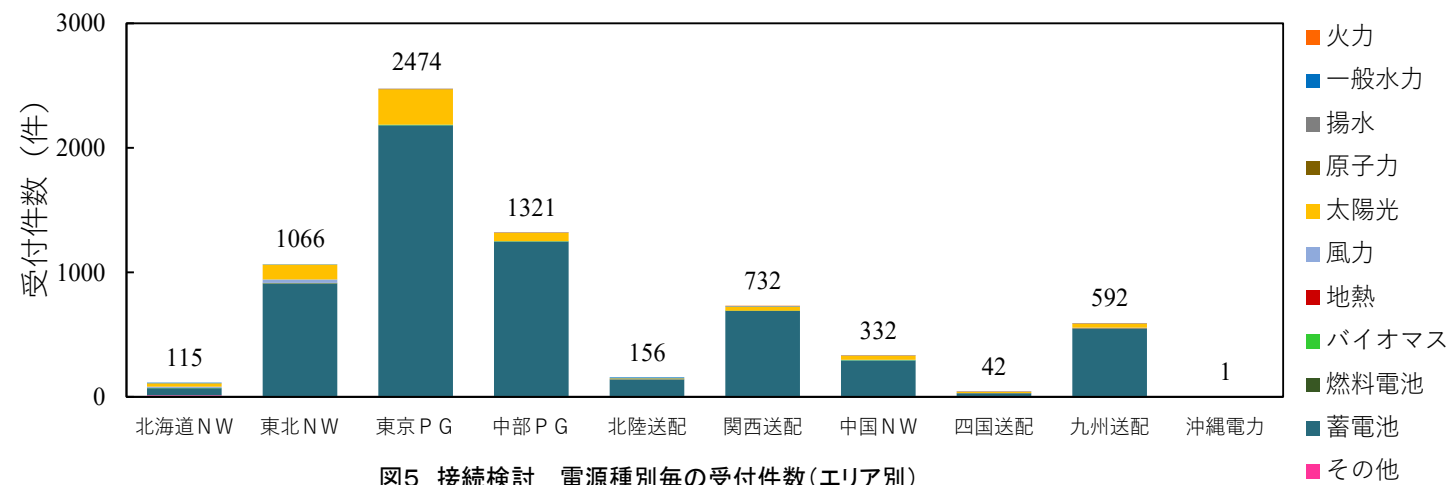
図5 接続検討 電源種別毎の受付件数(エリア別) [2026年度4月～6月]
