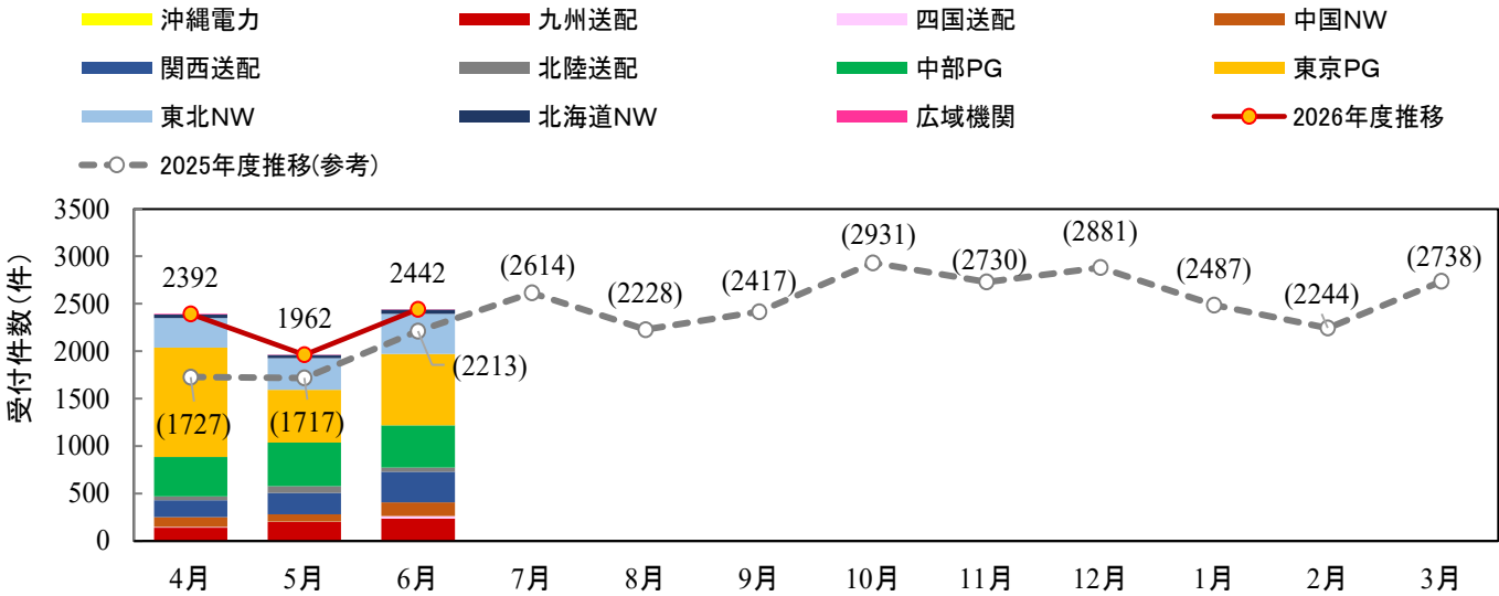
図4 接続検討 受付件数(広域機関＋一般送配電事業者合計) [2026年度4月～6月]
