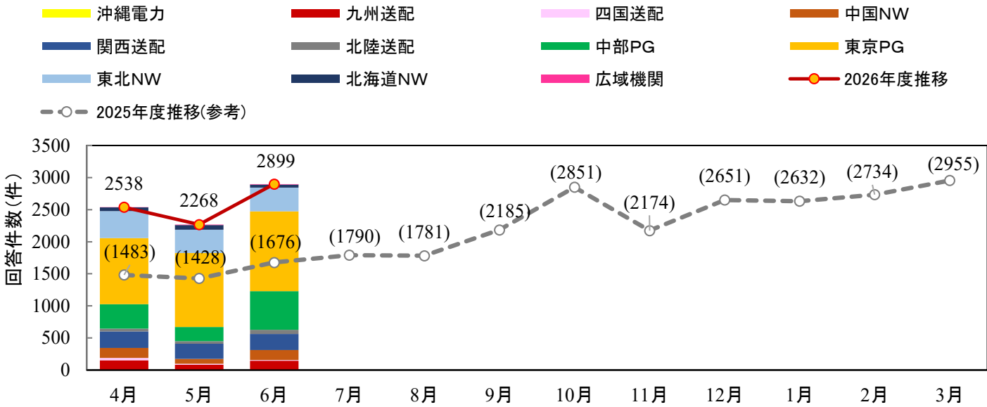
図9 接続検討 回答件数(広域機関＋一般送配電事業者合計) [2026年度4月～6月]
