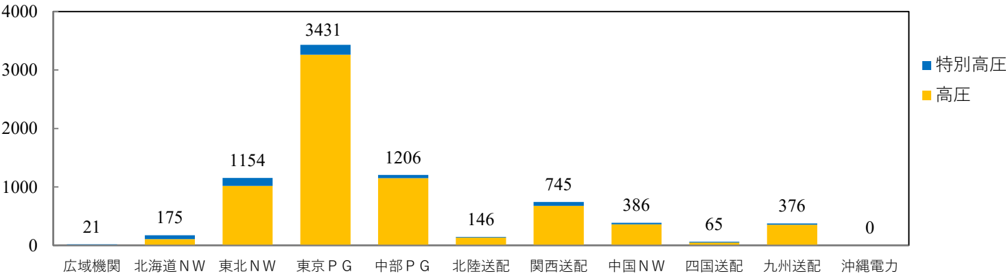
図8 接続検討 回答件数(広域機関および一般送配電事業者別) [2026年度4月～6月]
