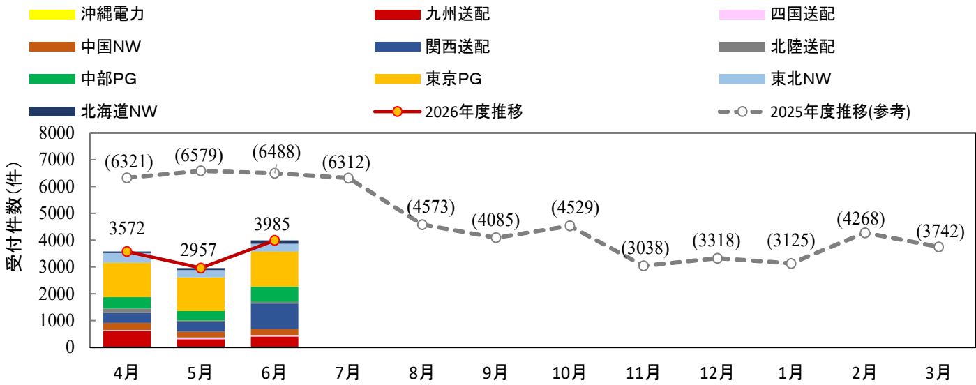
図2 事前相談 受付件数(一般送配電事業者合計) [2026年度4月～6月]
