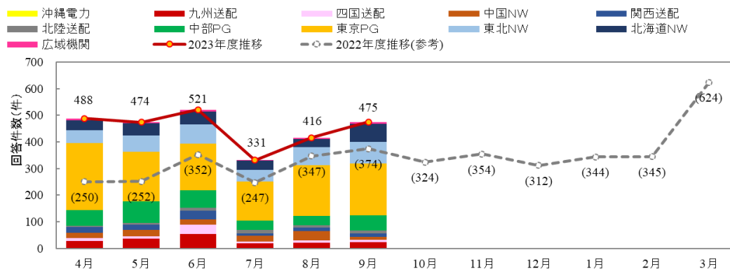
図9 接続検討 回答件数(広域機関+一般送配電事業者) [2023年度7～9月]
