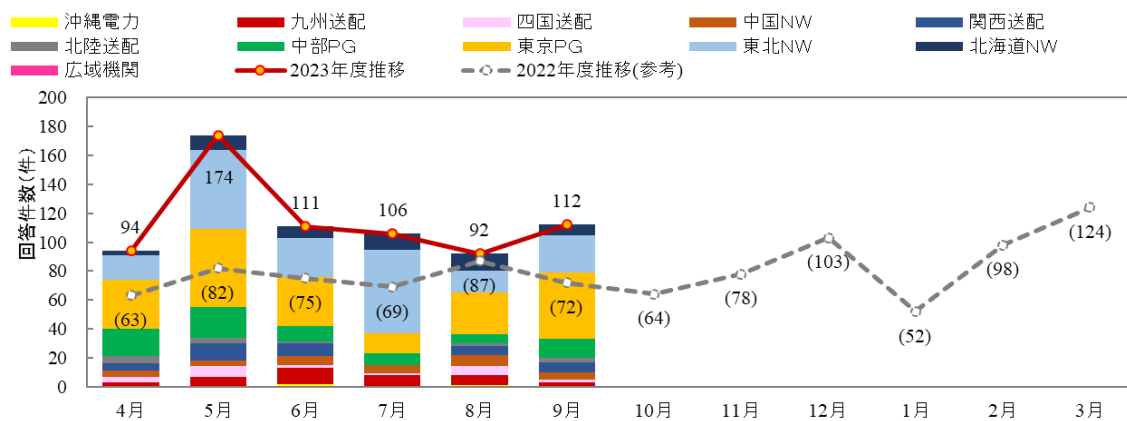
図19 契約申込み 回答件数(広域機関+一般送配電事業者) [2023年度7～9月]
