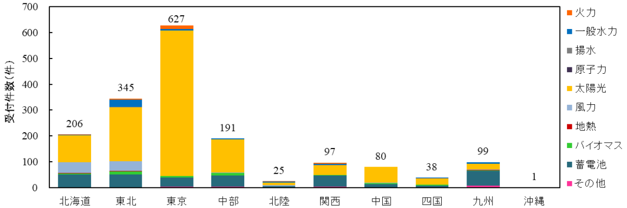
図5 接続検討 電源種別毎の受付件数(エリア別) [2023年度7～9月]
