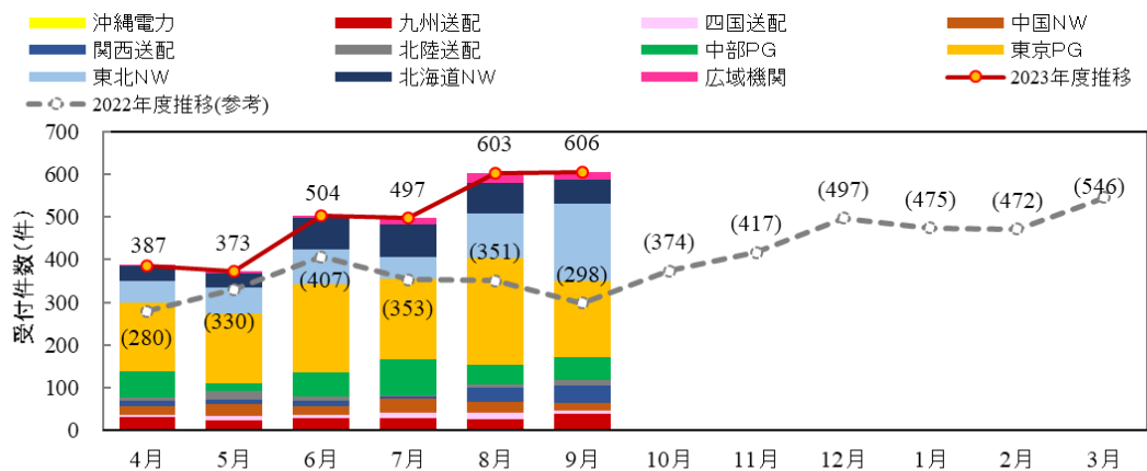
図4 接続検討 受付件数(広域機関+一般送配電事業者合計) [2023年度7～9月]
