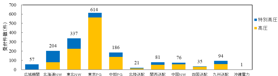
図3 接続検討 受付件数(広域機関および一般送配電事業者別) [2023年度7～9月]
