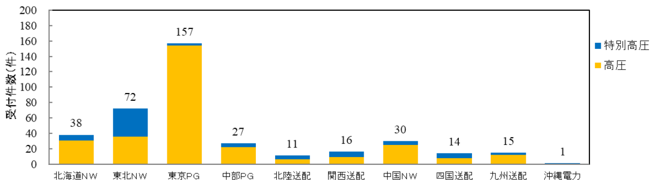
図13 契約申込み 受付件数(広域機関および一般送配電事業者別) [2023年度7～9月]
