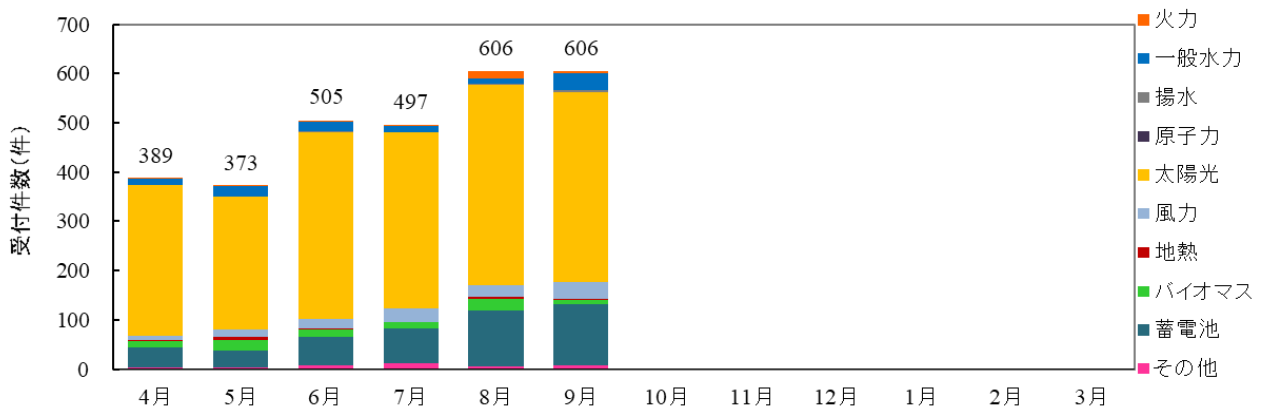
図6 接続検討 電源種別毎の受付件数(全エリア合計) [2023年度7～9月]
