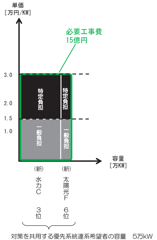
〔②その他供給設備工事 (110kV送電線増強工事) 〕
