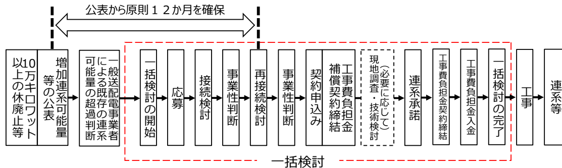
図6 一括検討のフロー（既存の連系可能量を超えると判断した場合）
