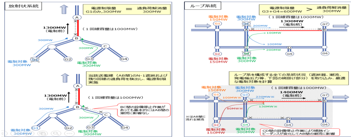
図 1－1 放射状系統とループ系統
