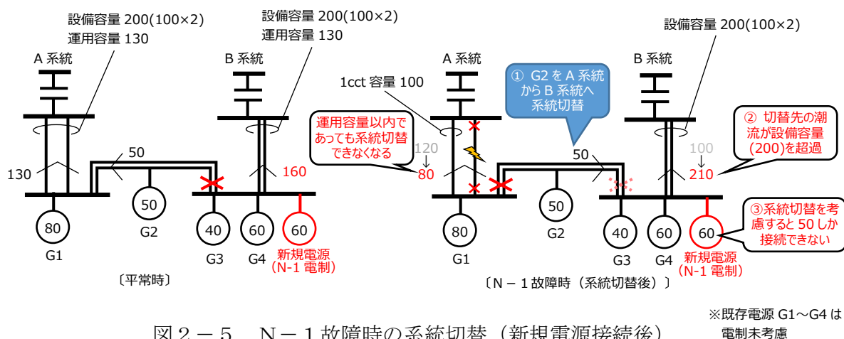
図2-5 N-1故障時の系統切替（新規電源接続後）
