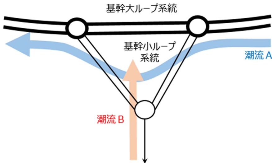
図 3－6 基幹小ループ系統の潮流
