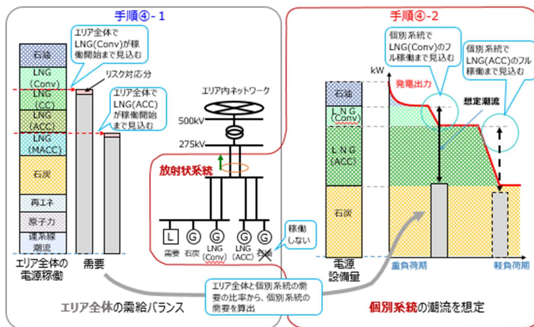
図 3-3 個別系統の潮流想定イメージ
