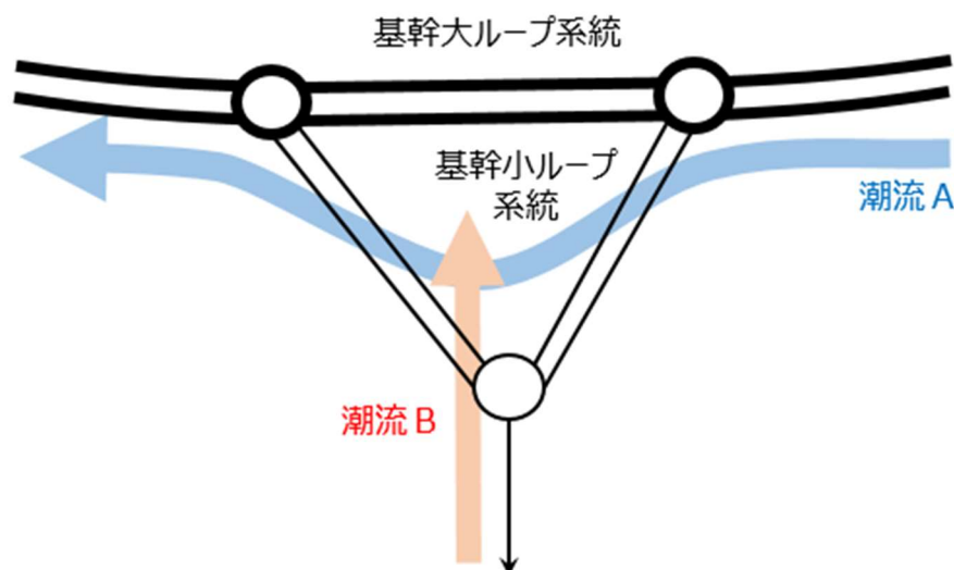
図2-1 基幹小ループ系統の潮流
