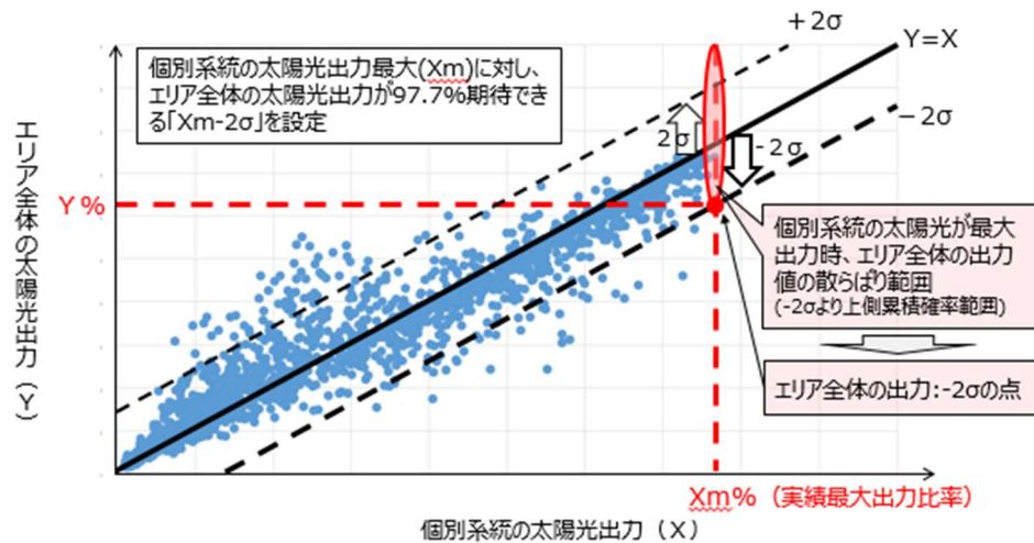
図3-2 エリア全体の太陽光出力と個別系統の太陽光出力との相関関係（イメージ図）
