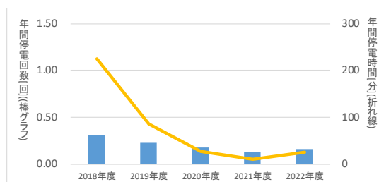
図19 (全国、2017～2021年度)低圧電灯需要家停電実績
