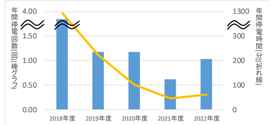
図29 (沖縄、2017～2021年度) 低圧電灯需要家停電実績
