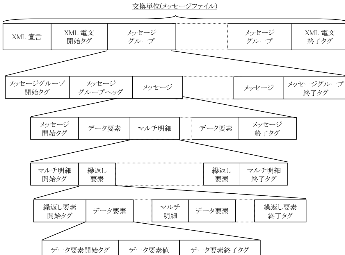
図 3-1 XML 電文の階層構造
